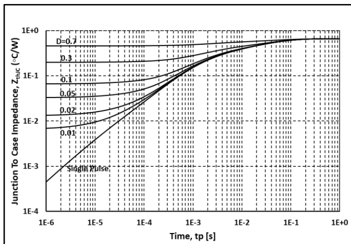
图. 25 热阻曲线
