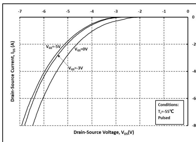
图. 10 体二极管导通曲线 @ T_J = -55°C
