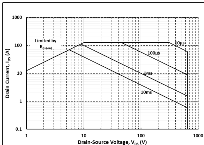
图. 26 安全工作区示意图
